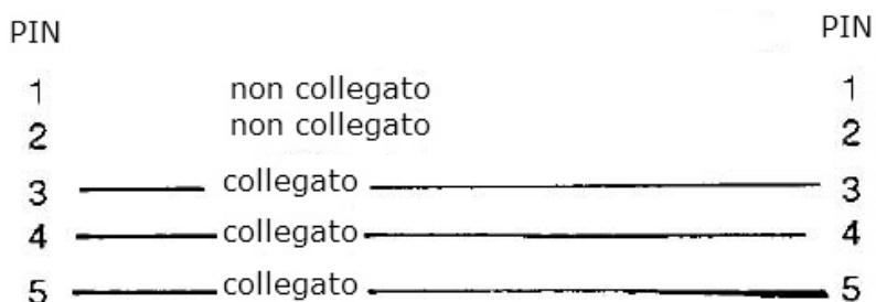
Spina Sensore / Attore 5 Poli
