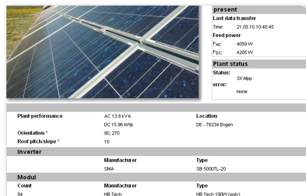
Dati dell'impianto nel Solar-Log™ WEB
