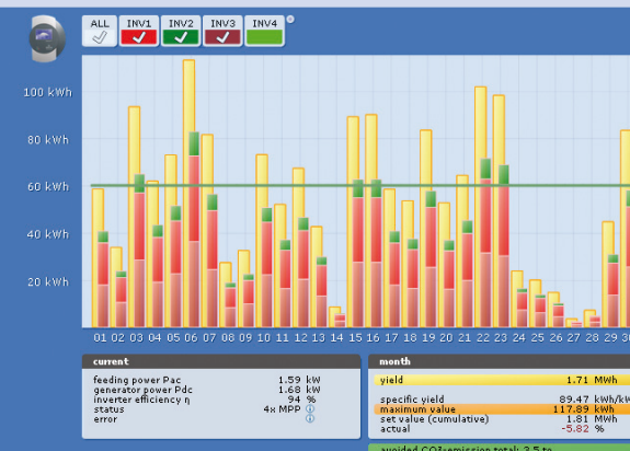
Solar-Log™ WEB – dati di produzione con parecchi inverter
